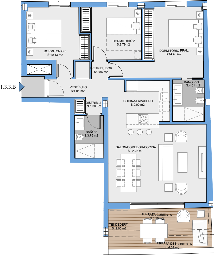
PLANTA SEGUNDA
